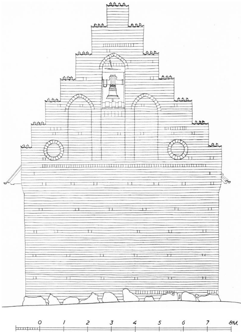
Fig. 5. Olstrup. Skibets vestgavl. 1:100. Målt af Jacob Blegvad 1944 (s. 707).
