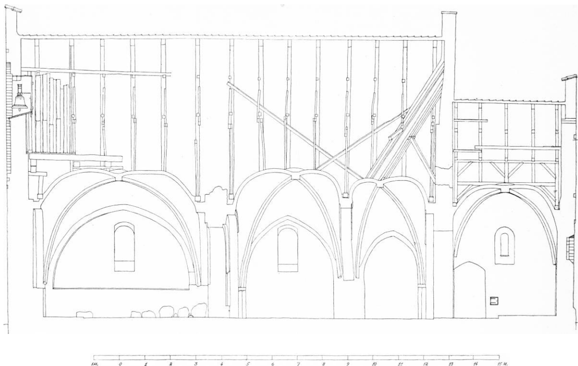
Fig. 4. Olstrup. Snit vest-ost. 1:150. Målt af Aage Andreasen 1944.
