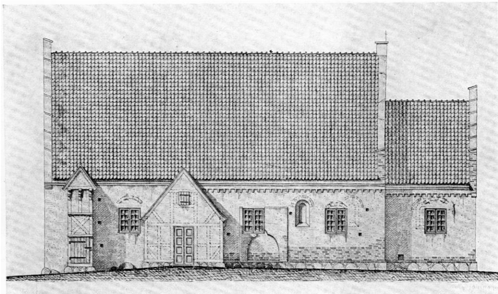
Fig. 3. Olstrup. Sydfaçade for restaureringen. 1:200. Målt af H. C. Glahn 1898.
