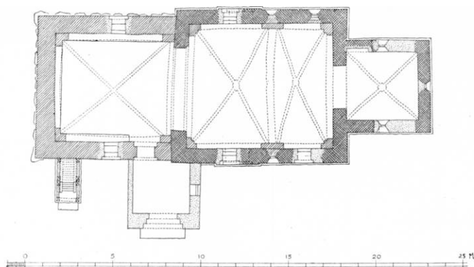
Fig. 2. Olstrup. Plan. 1:300. Målt af Mogens Windfeldt Jensen 1944.
