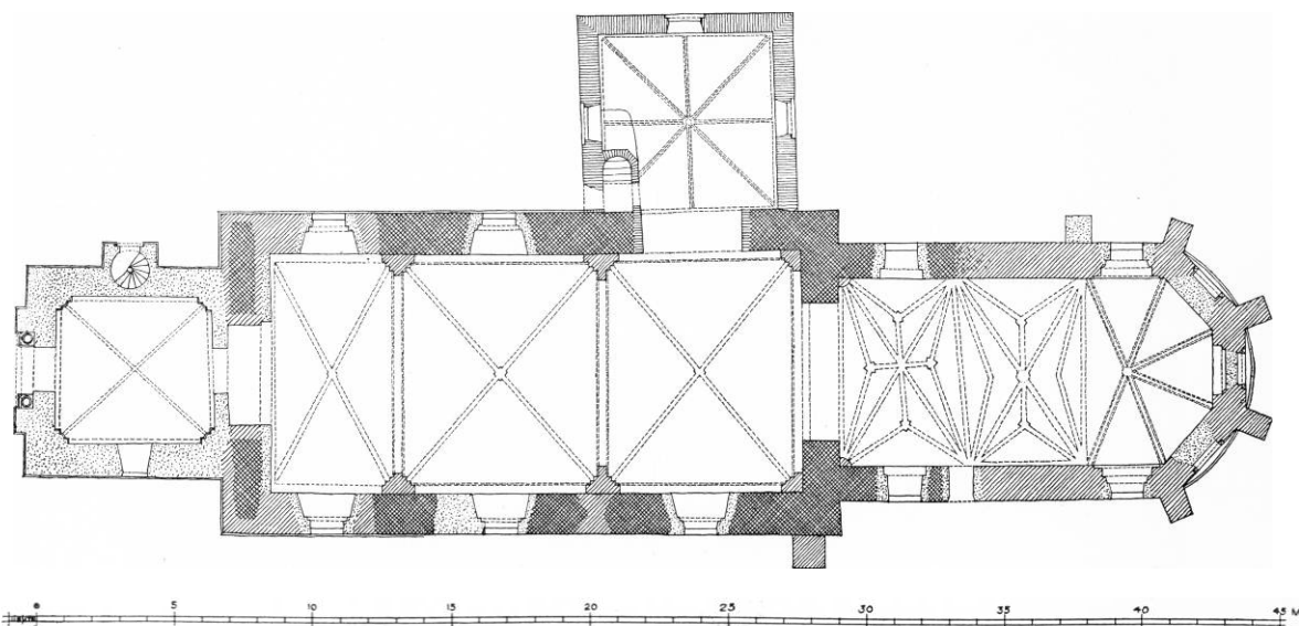
Fig. 2. Halsted. Plan. 1:300. Målt af C. G. S. 1948.
