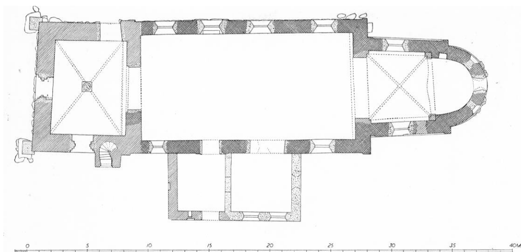
Fig. 2. Horslunde. Plan. 1:300. Målt af A. W. Fyhn 1951.
