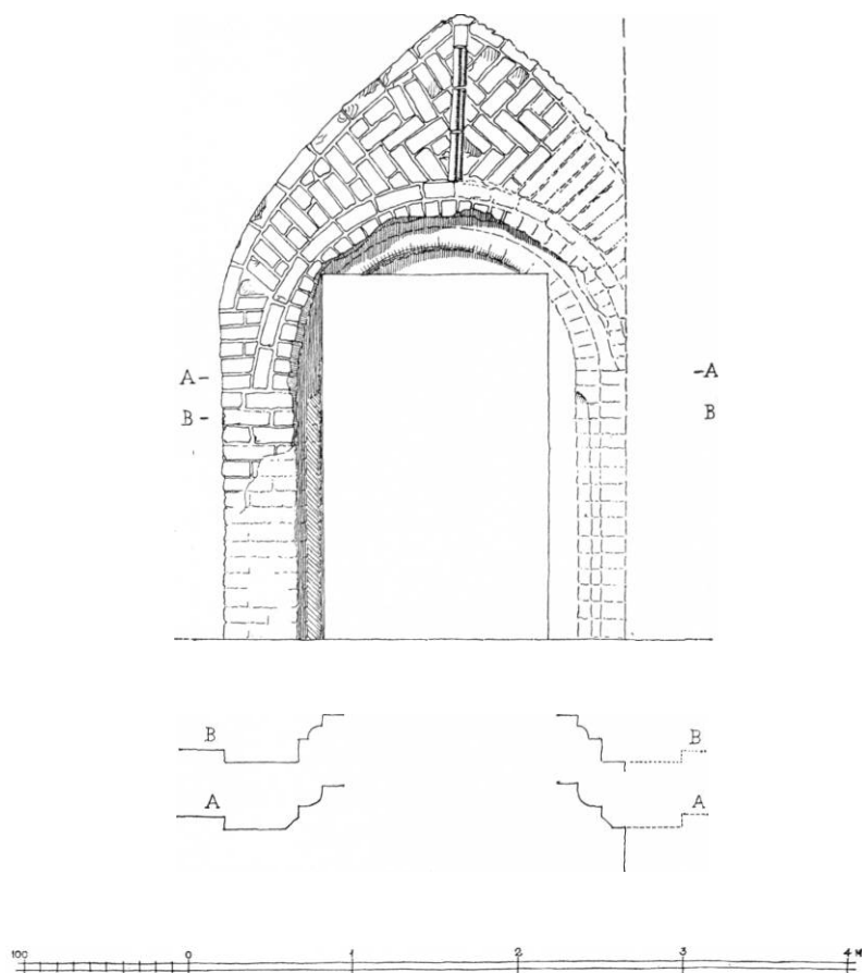
Fig. 5. Horslunde. Sydportal. 1:50. Målt af Charles Christensen 1950 (s. 548).
