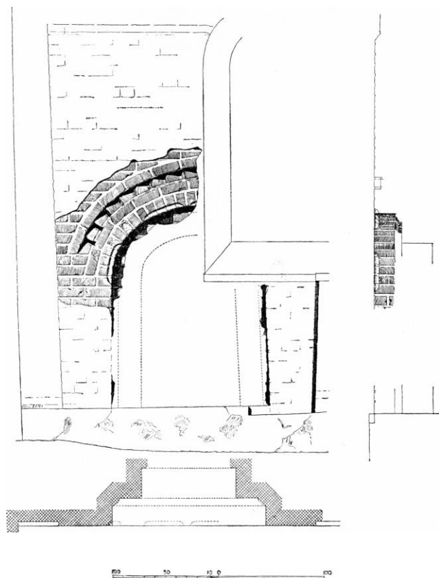
Fig. 4. Horslunde. Præstedor i korets sydside. 1:50. Målt af Per Molnit 1941 (s. 548).
