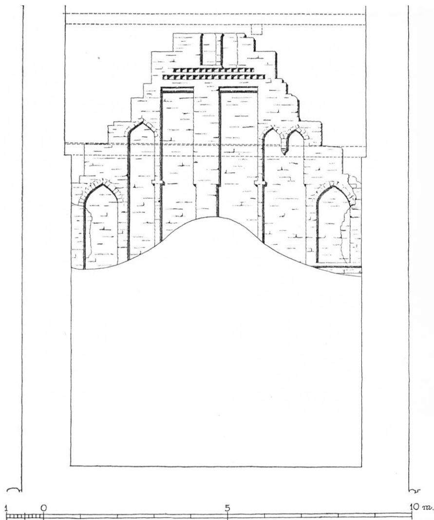
Fig. 6. Horslunde. Skibets vestgavl. 1:100. Målt af Per Molnit 1941 (s. 549).
