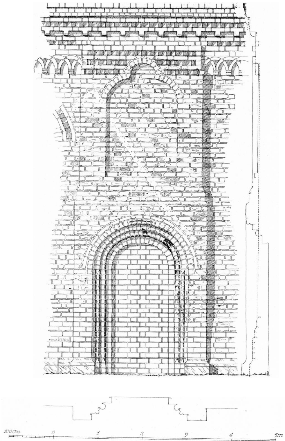
Fig. 7. Saksøbing. Nordportal. Målt af Aa. Rl. 1944.
