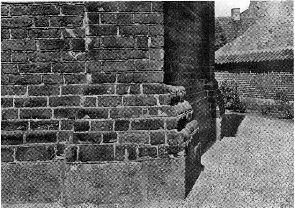
Fig. 5. Sakskøbing. Apsissokkel (s. 132).
