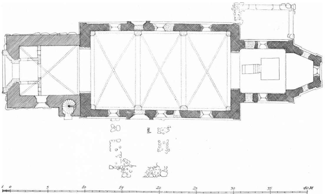
Fig. 3. Sakskøbing. Plan. 1:300. Målt af J. og H.Hansen 1944 (Aa. RI. 1945).
