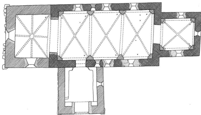
Fig.2-3. Plan 1:300 og tværsnit af skib 1:150. Målt af E1M 1966, tegnet af Flemming Beyer 1980. - Groundplan 1:300 and cross-section of nave 1:150.
