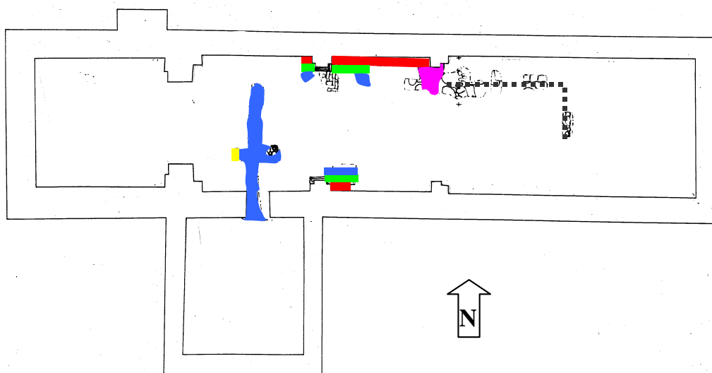
Fig. 3. Grundplan af Skamstrup kirke med indtegnede udgravningsfelter (grøfter til varmerør). Rød: vægbænk, grøn: fodtrin, blå: mørtelgulv, gul: hævet podium i skibets vestligste del, lilla: fundament fra oprindelig triumfmur, stiplet: inderside af mur i det tidligere (og mindre) kor.
